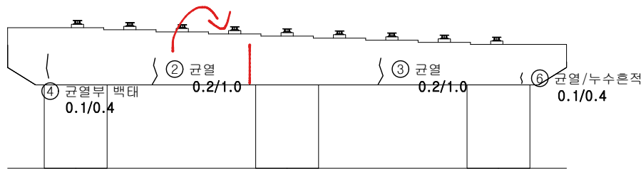
배면
